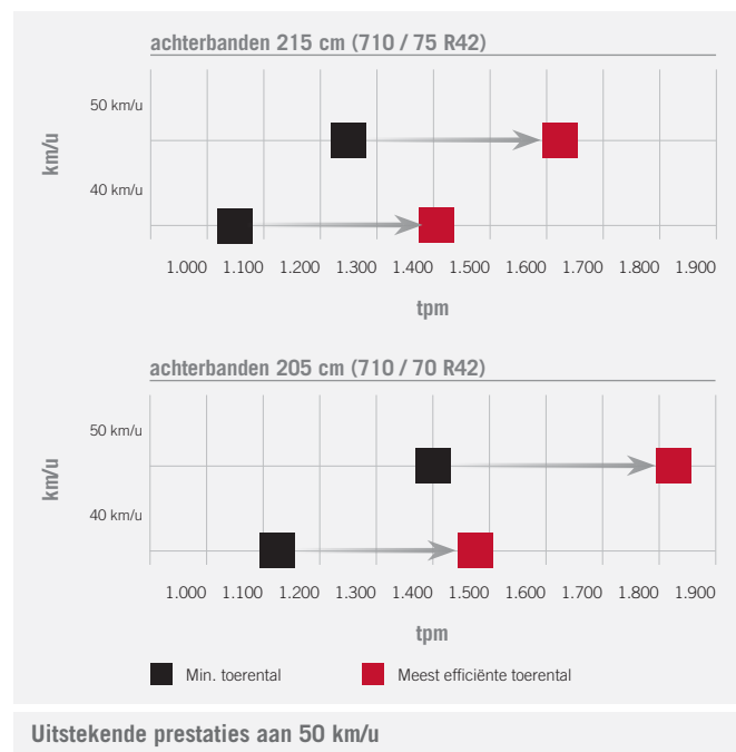
CVX-transmissie - traploze aandrijving tussen 0 en 50 km/u
