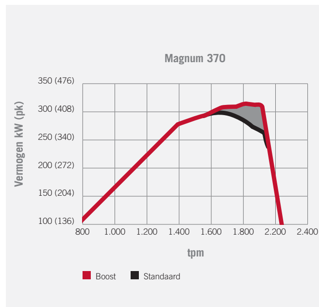
35 pk extra met vermogensboost
